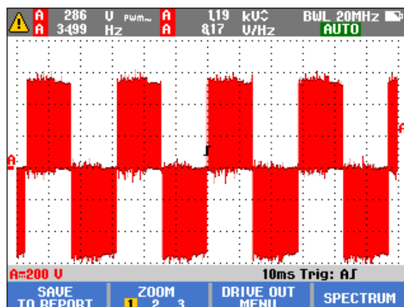
드라이브 출력 파형 자동 트리거
