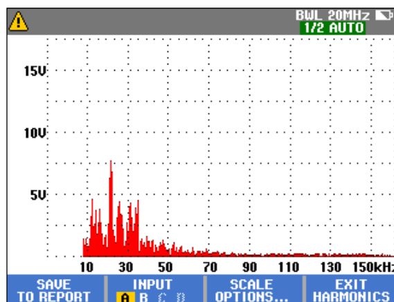
9kHz에서 150kHz로 확장된 고조파 스펙트럼
