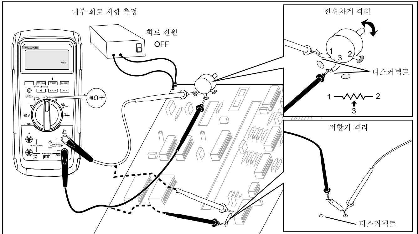
그림 5. 저항 측정
