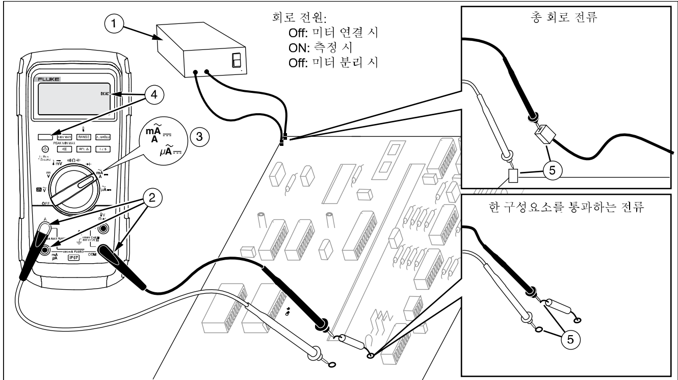
그림 8. 전류 측정
