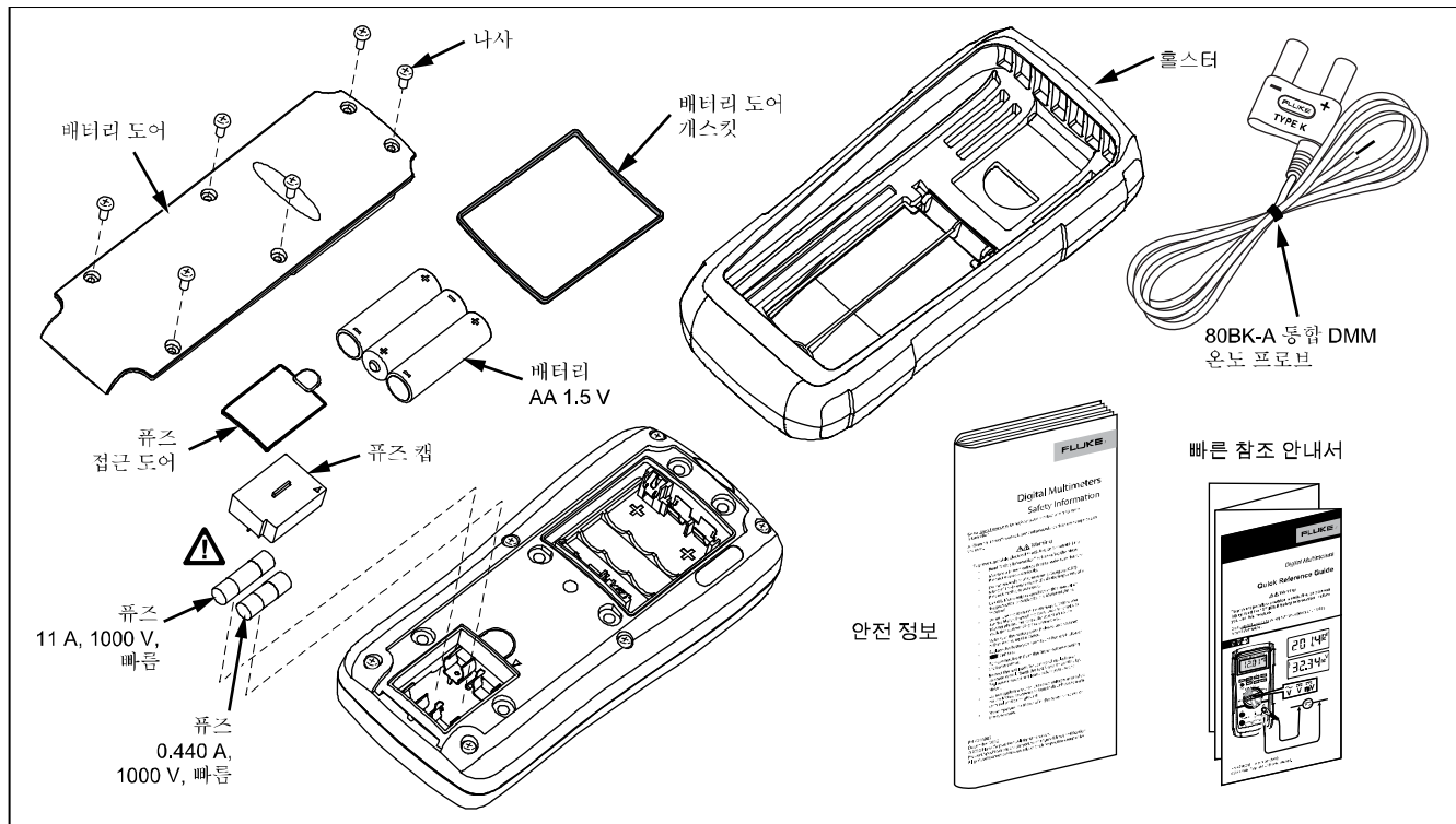
그림 12. 교체 부품
