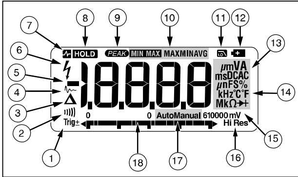
그림 1. 디스플레이 기능
