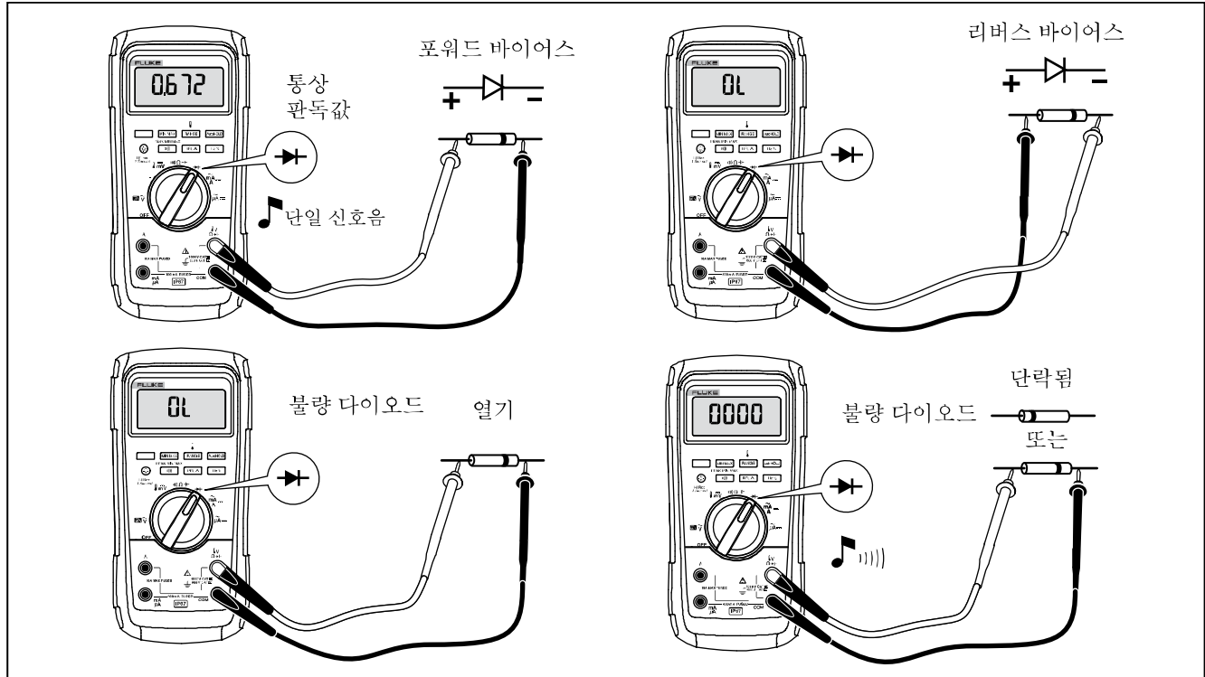
그림 7. 다이오드 테스트
