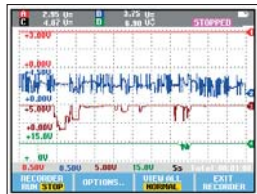
Fluke 190 시리즈 II의 커서 및 줌 기능을 사용해 캡처된 TrendPlot을 분석할 수 있습니다.
