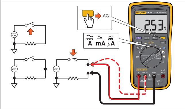
그림 4.AC 또는 DC 전류 측정
