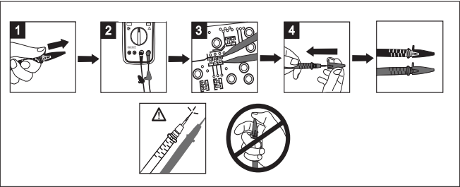
그림 9. 회로의 작은 구성 요소 테스트
