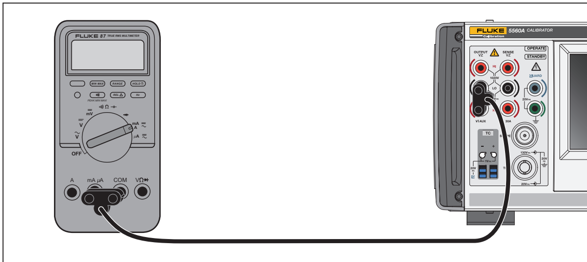
그림 7.DUT 연결 : DC 전류 /AC 전류 < 3.1A
