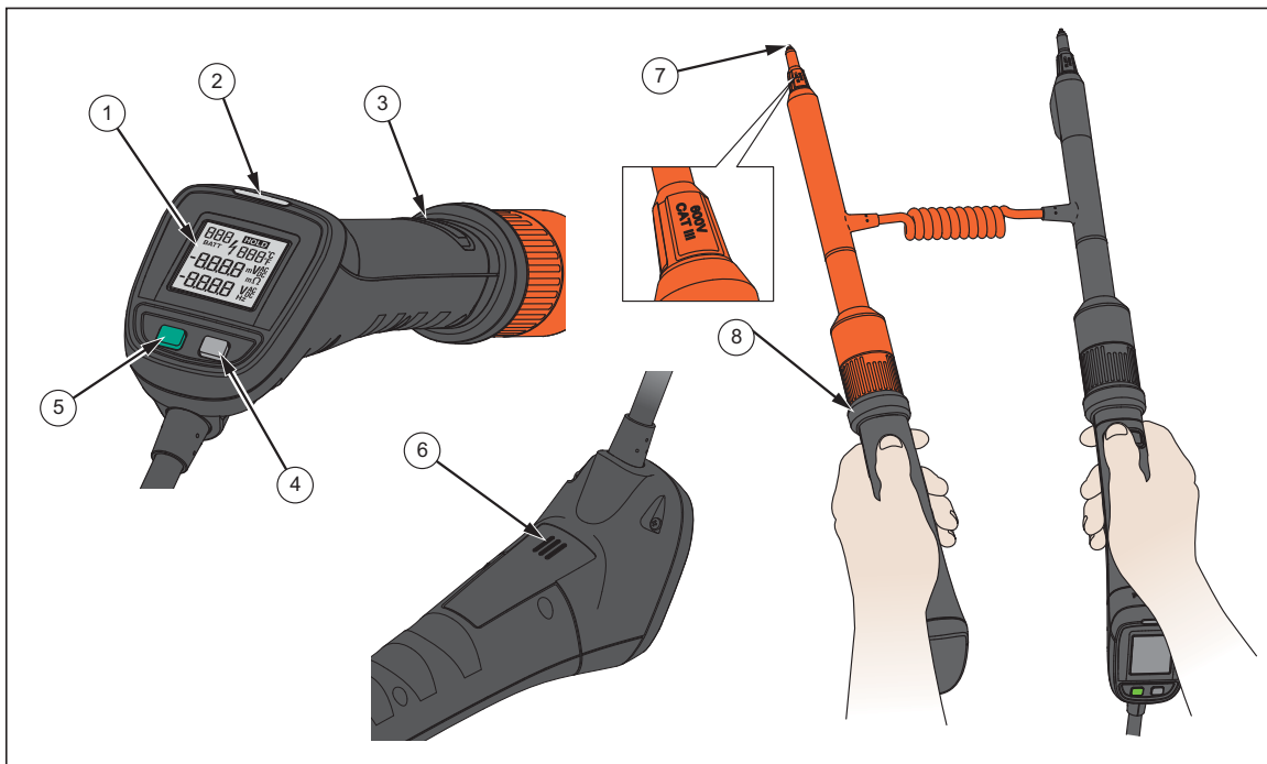
그림 4-1. BTL21 Interactive Test Probe
