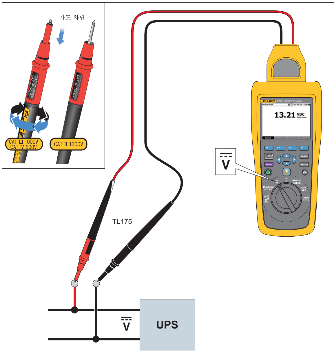
그림 3-6. TL175 를 사용한 DC 전압 측정
