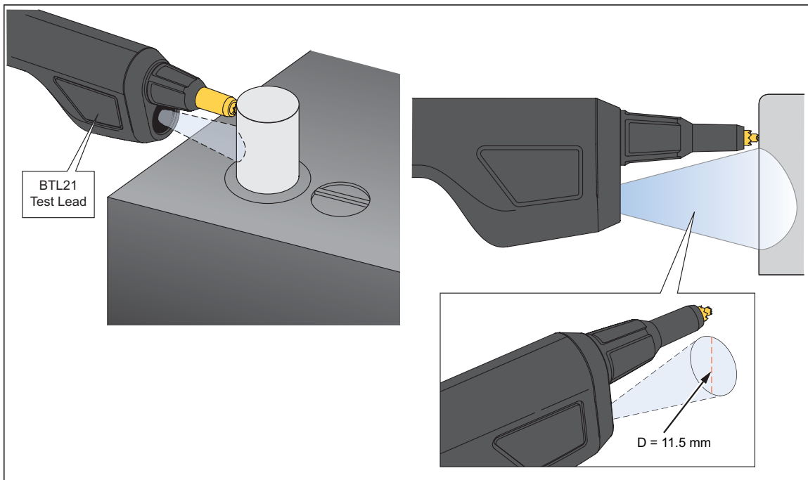
그림 4-6. 배터리 극의 온도 측정
