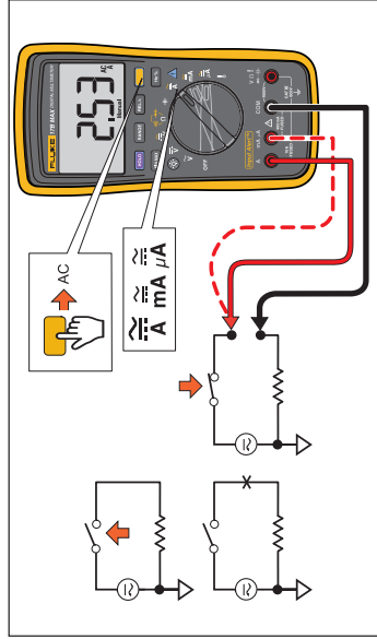
그림 4.AC 또는 DC 전류 측정
