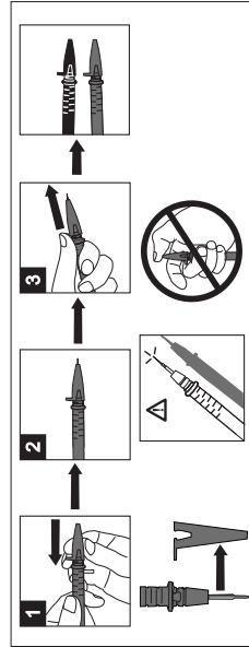
그림 10. CAT III 애플리케이션을 위한 프로브 위치
