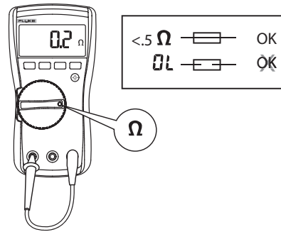
그림 1. 퓨즈 테스트
