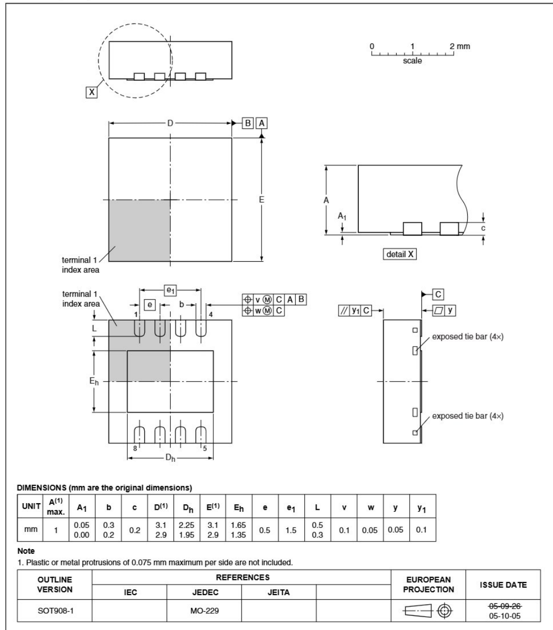
Fig 18. Package outline SOT908-1 (HVSON8)
