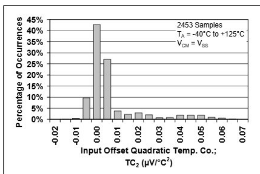
FIGURE 2-3: Input Offset Quadratic Temp. Co.
