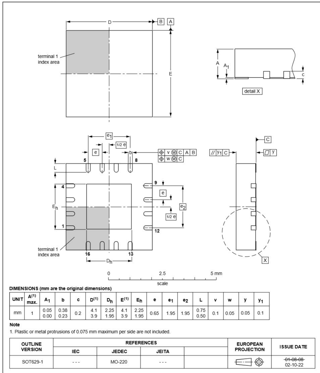
Fig 30. Package outline SOT629-1 (HVQFN16)
