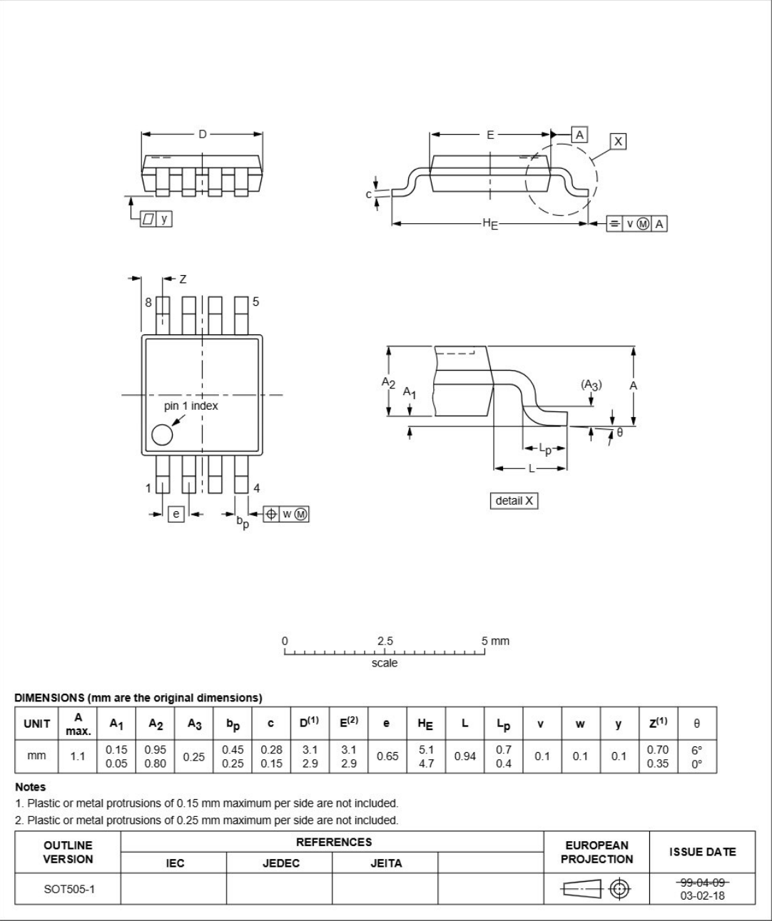
Fig 27. Package outline SOT505-1 (TSSOP8)
